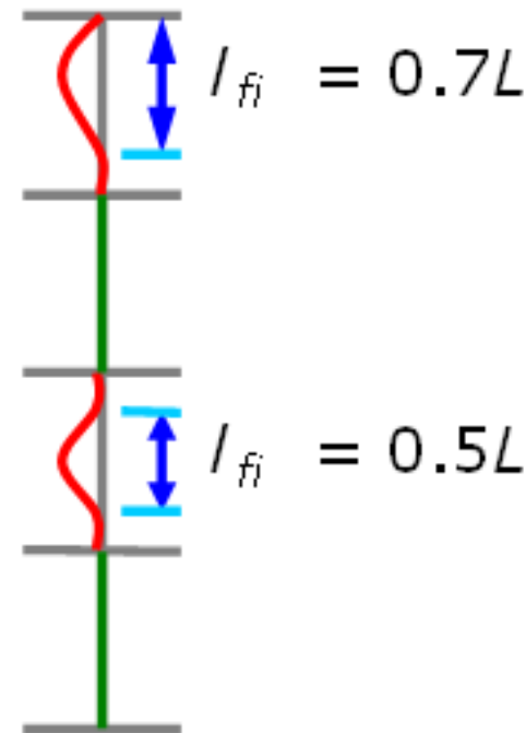
Kihajlási alak tűzhatás esetén
