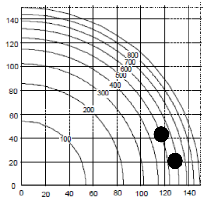
A17. ábra: Hőmérséklet-eloszlás (°C) kör keresztmetszetű oszlopban, d = 300 mm, R 60
